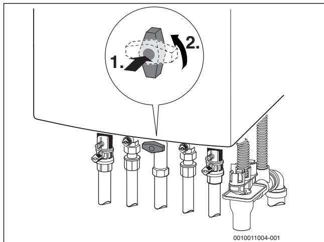
Фиг. 2 Отваряне на газовия кран
